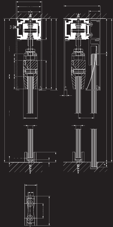
Kosi-D für Wand-/ Deckenmontage (mit und ohne Verkleidungsprofil)
